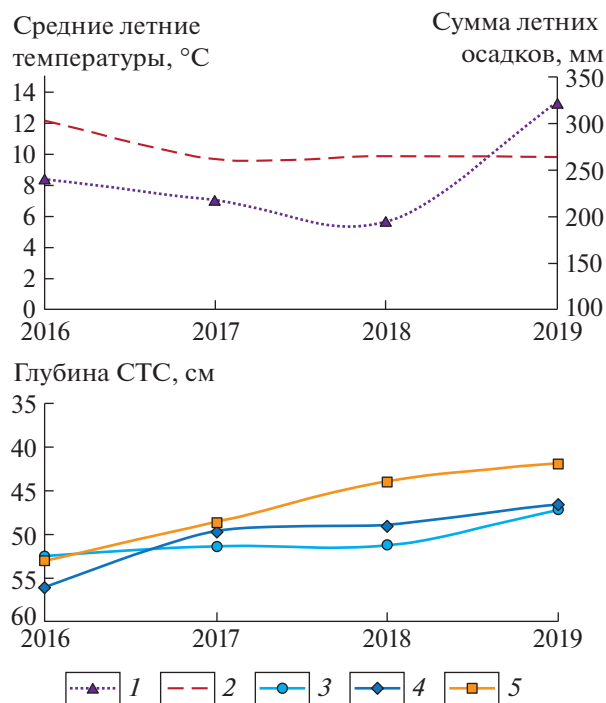
Рис. 2. Глубина СТС на разных элементах микро-рельефа торфяника 1. 1 – сумма летних осадков; 2 – средние летние температуры воздуха; Глубина СТС: 3 – в центральной части полигонов; 4 – в периферийной части полигонов; 5 – в межполигональных понижениях.
